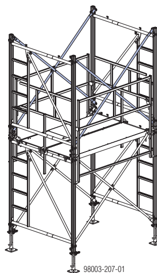
F Диагонална X-връзка
