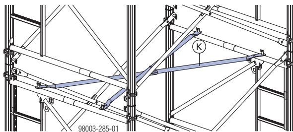
K Диагонална X-връзка
