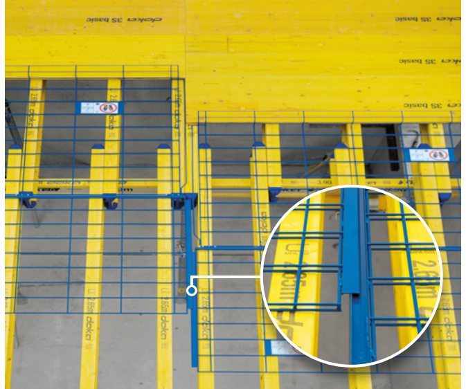
Safeflex-Schiebegitter mit Führungsschiene
