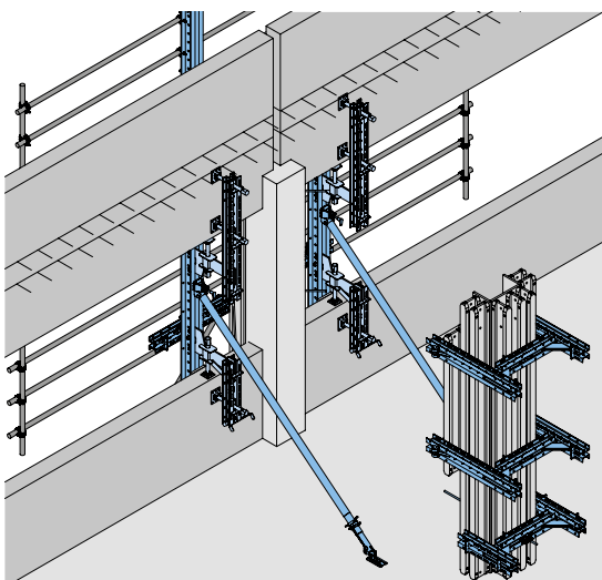
Integrierte und zurückgesetzte Ortbetonstützen: Sowohl bei integrierten Ortbetonstützen als auch bei zurückgesetzten Ortbetonstützen ist die Fassadenschalung Top 50 die wirtschaftliche Lösung bei Bauvorhaben mit Fertigteilfassaden.
