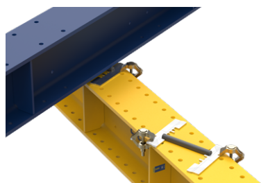
Dumanja Jaruga | Kroatien | Doka UniKit Lastturm 480kN, Joch- und Längsträger, Verlängerungen und Schwerlastjochs
