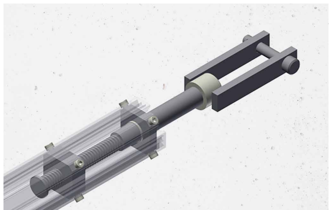
Das verdeckte Gewinde schützt vor Verschmutzung und sorgt für hohe Langlebigkeit und geringen Wartungsaufwand.
