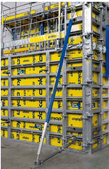
Elementstütze an der Schalung (mit Elementstützenschuh)
