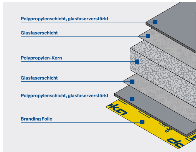
Aufbau Xlife top Platte
