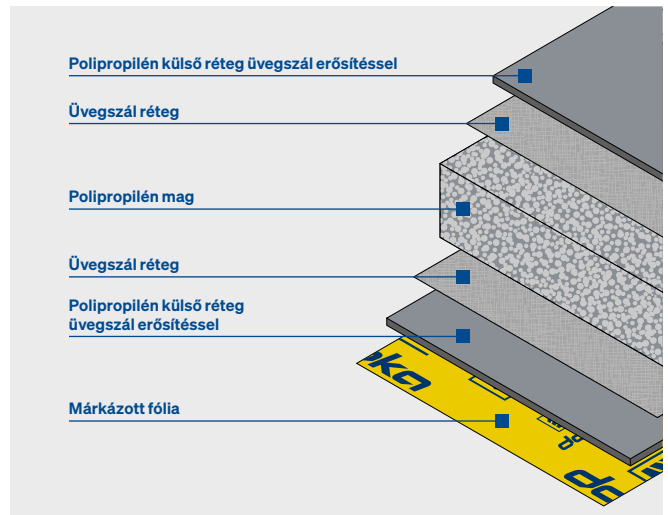
Az Xlife top zsaluhéj szerkezete
