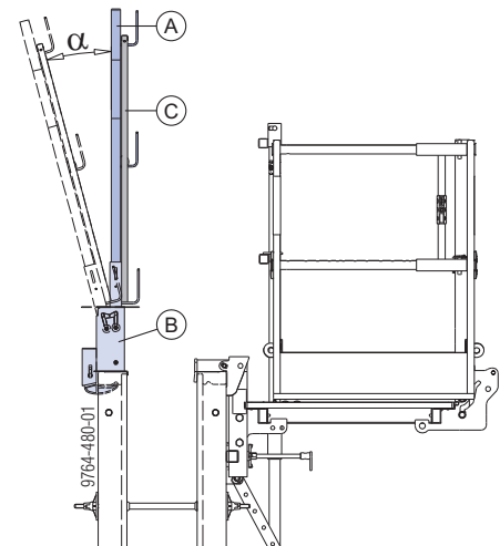
A עמוד מעקה XP 1.20 מ'
