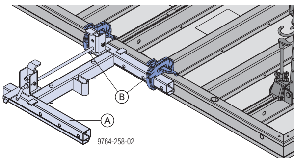
A תבנית טפסות קיר של מחבר XS
