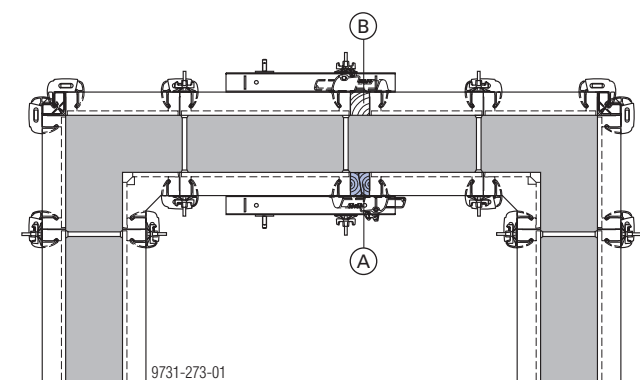
A פנימי - עץ פירוק B חיצוני - עץ חיבור
