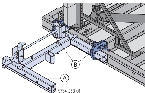
A תבנית טפסות קיר של מחבר XS
