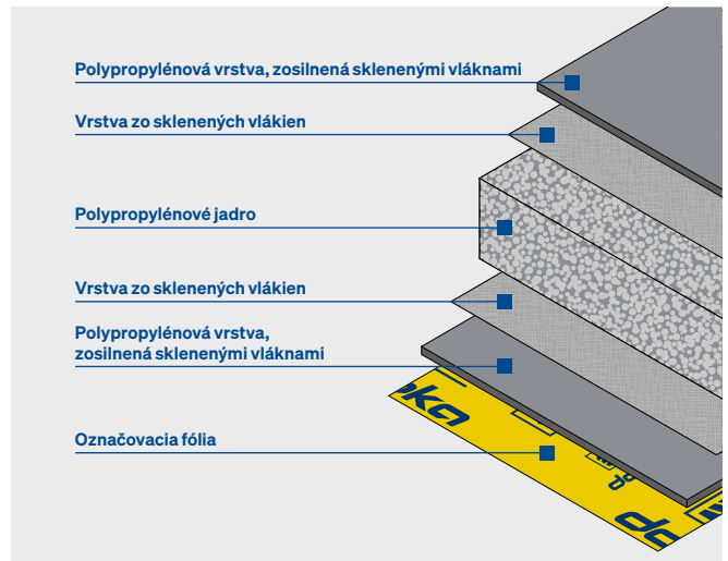
Konštrukcia dosky Xlife top
