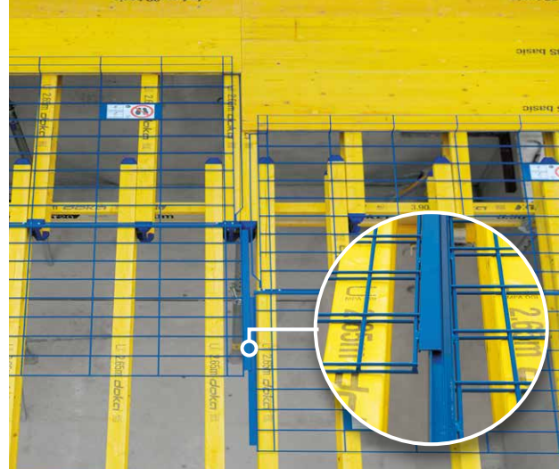
Grille coulissante Safeflex avec rail de guidage
