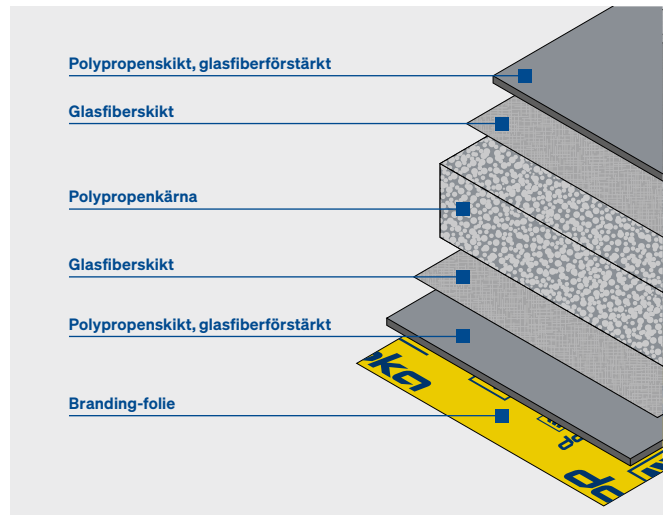
Xlife top-formskivans uppbyggnad
