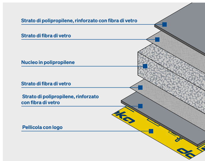
Struttura del pannello Xlife top
