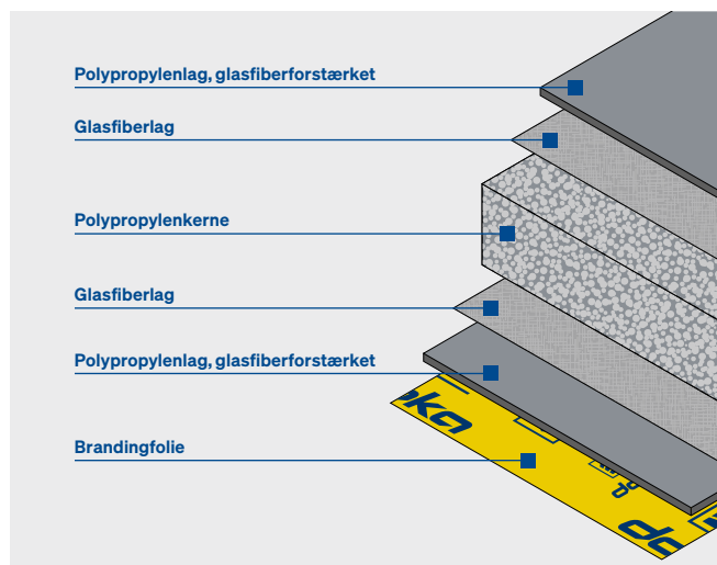
Xlife-toppladens struktur
