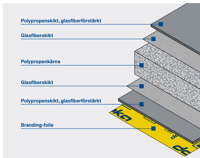
Xlife top-formskivans uppbyggnad
