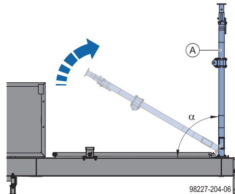
A Doka-Deckenstütze
