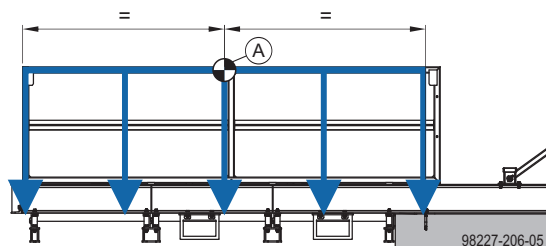
A Lastschwerpunkt
