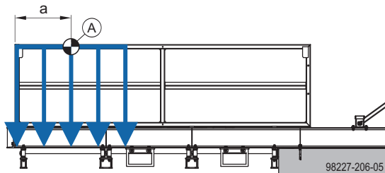
A Lastschwerpunkt
