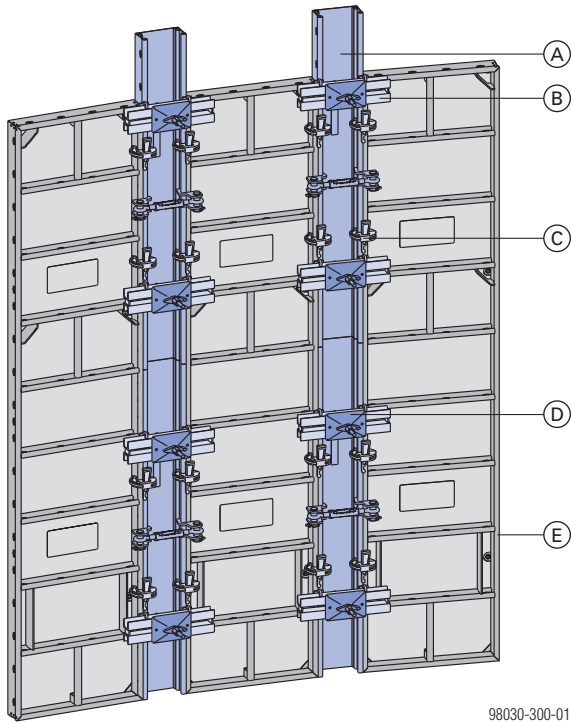
Darstellung mit Frami Xlife-Element 2,70m.
