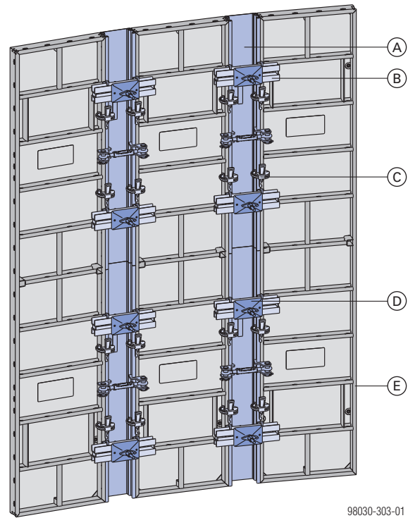
Darstellung mit Frami Xlife-Element 3,00m.
