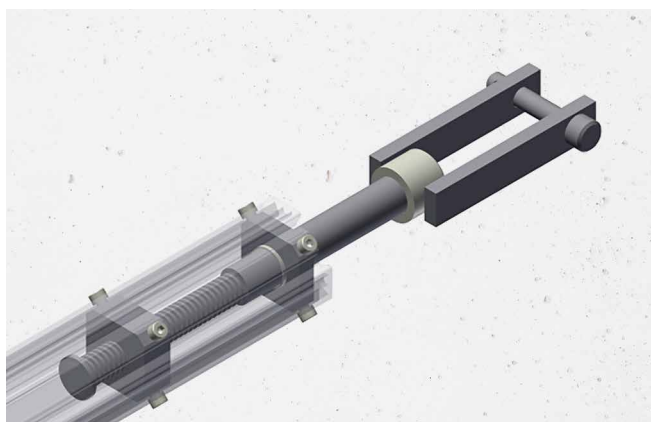
A kialakítás miatt a belső menet védett a szennyeződéssel szemben. Ez nemcsak a termék élettartamát hosszabbítja meg, de a karbantartás gyakoriságát is csökkenti.
