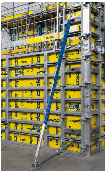
Beállító támasz a zsalun (zsaluadapter csapszeg szettel)
