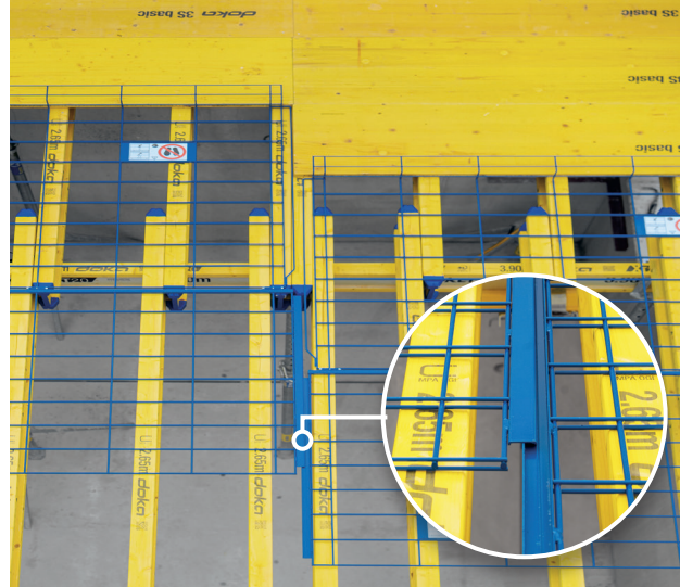
Grille coulissante Safeflex avec rail de guidage
