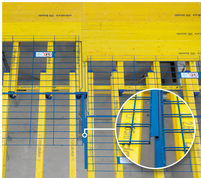
Grille coulissante Safeflex avec rail de guidage
