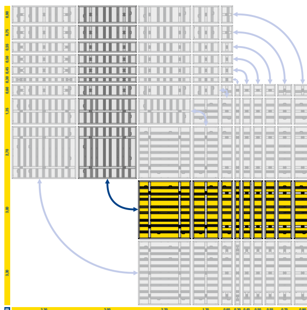
Hauteur de panneau 3,00 m : horizontale et verticale, peut être combiné avec toutes les hauteurs de système
