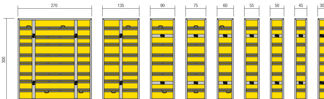
Combinaison des panneaux de Framax Xlife plus 3,00 m / Indications en cm
