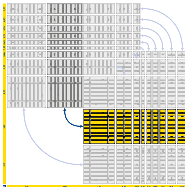
3-meters luckan kan kombineras liggande och stående med alla systemhöjder
