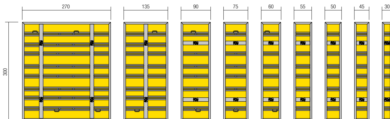
Luckmått för Framax Xlife plus 3,00 m / uppgifter i cm
