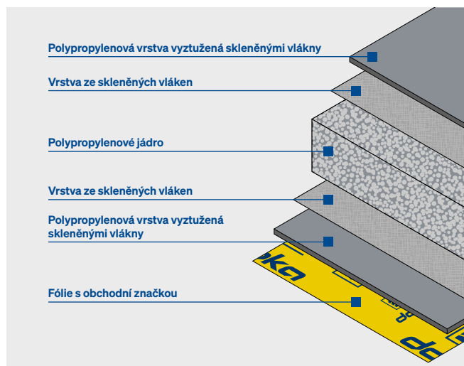
Struktura bednicí desky Xlife top
