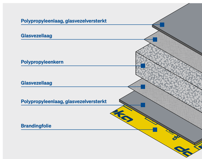
Opbouw Xlife top plaat
