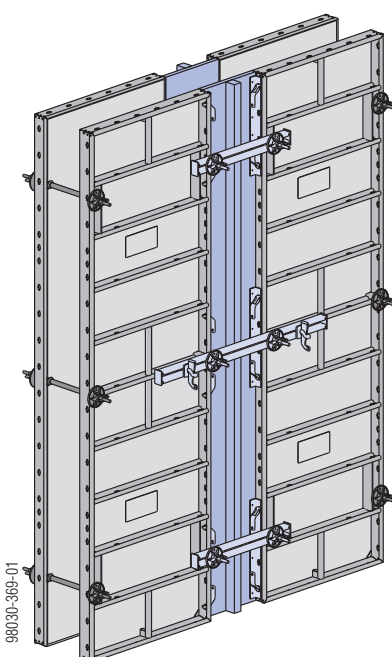
Illustrazione con elemento Frami Xlife 3,00m.
