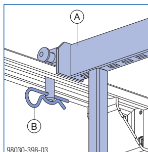
Protezione contro lo scardinamento
