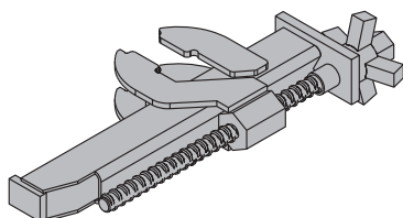
Morsetto di compensazione Frami: forza di trazione ammessa: 7,5 kN
