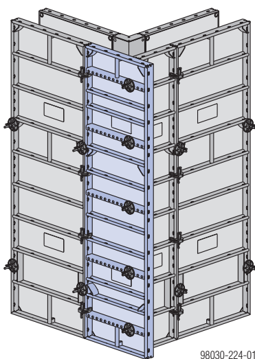
Illustrazione con elemento Frami Xlife 2,70m.
