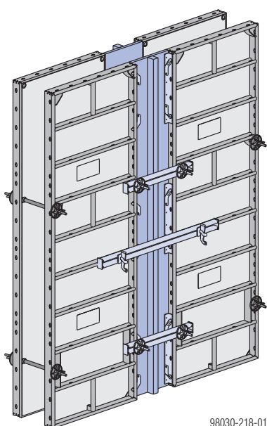
Illustrazione con elemento Frami Xlife 2,70m.
