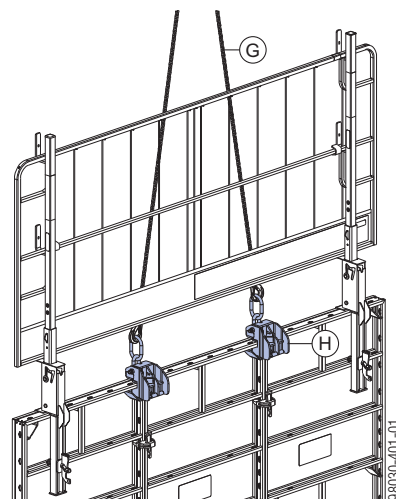
G Catena di sospensione a 4 funi Doka
