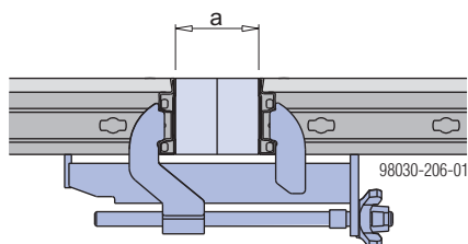
Morsetto di compensazione Frami: forza di trazione ammessa: 7,5 kN
