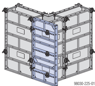
Illustrazione con elemento Frami Xlife 1,50m.
