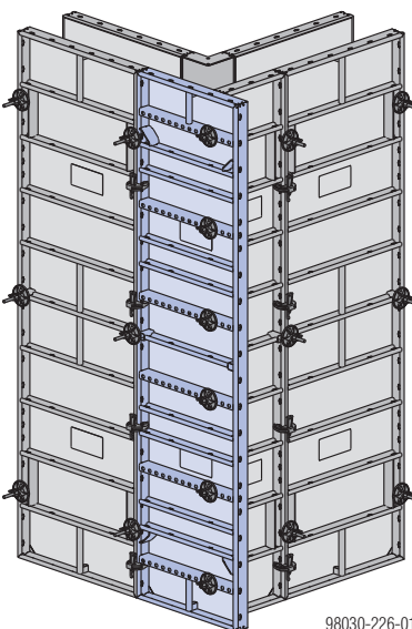
Illustrazione con elemento Frami Xlife 3,00m.
