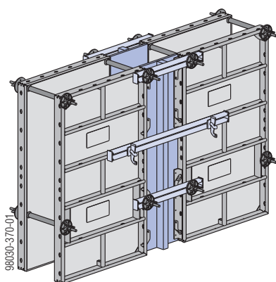
Illustrazione con elemento Frami Xlife 1,50m.
