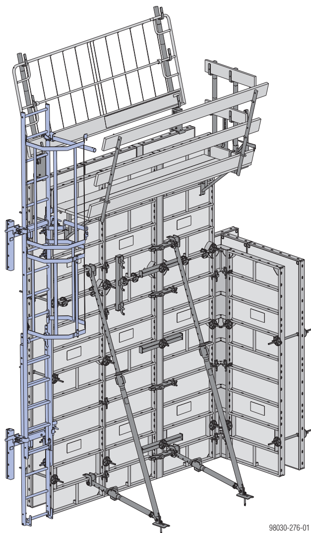
Illustrazione con elemento Frami Xlife 2,70 m.
