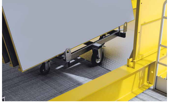
Die Auffahrrampe gewährleistet das sichere und leichtgängige Überfahren der Bauwerkskante.
