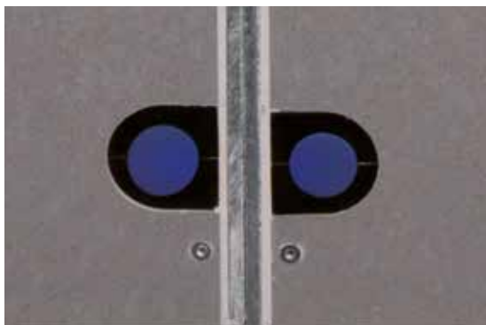
Az ankerrudak átvezetése során a tartós Xlife zsaluhéjat az integrált ankervédők kímélik meg ez esetleges sérülésektől
