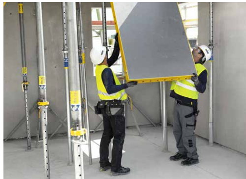
Le coffrage modulaire de dalles DokaXdek est un système de panneau flexible et léger pour une équipe de deux coffreurs.
