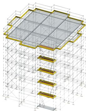
Schelă multidirecțională
