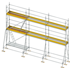
Schelă pentru armătură
