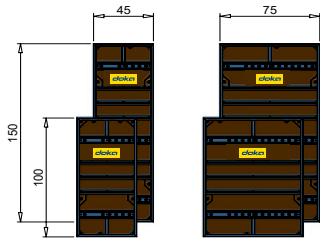
Kolonlar için 5 cm ızgaralı evrensel paneller
