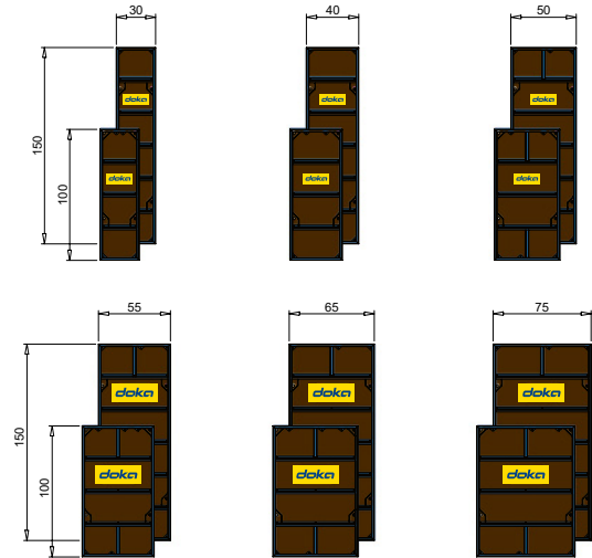
Mükemmel uygulanabilirlik için 5 cm aralıklı sistem ızgaralı standart paneller
