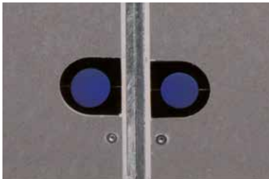
Integroitu ankkurisuoja ehkäisee tukevan Xlife-levyn vaurioitumisen ankkuritankoa sisään pujotettaessa.
