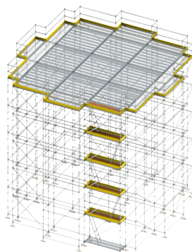
Rusztowanie przestrzenne
