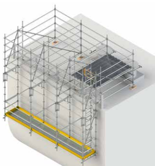
Rusztowanie podwieszane
