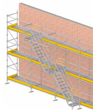
Rusztowanie elewacyjne
