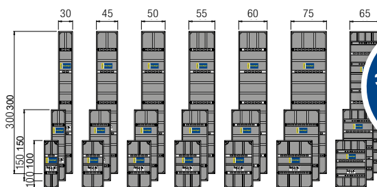
Einfache Anpassung an das Bauwerk durch praxisingerechtes Elementraster
