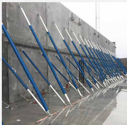
På betonelementer
