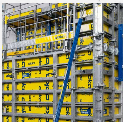
Formstøtter på forskalling (med formstøttehoved og formadaptersko)
