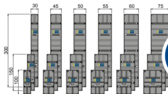
Einfache Anpassung an das Bauwerk durch praxismgerechten Elementraster
