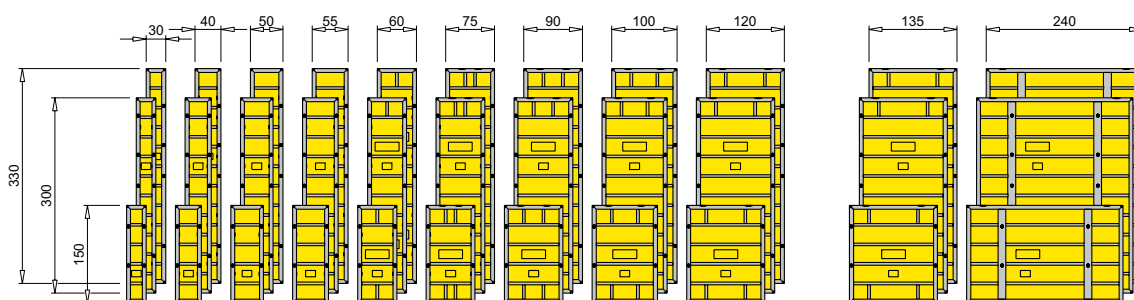
Размеры щитов ReForma Standard plus в см (щиты шириной 135 и 240 см изготавливаются под заказ)
