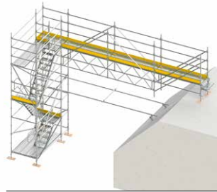
Ülekäigutellingud
