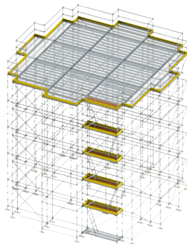
Linnupuurtellingud
