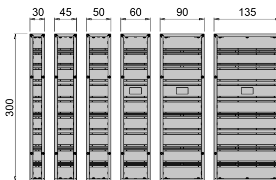
Podstawowe formaty paneli zostały zoptymalizowane pod kątem deskowania ścian budynków mieszkalnych.
