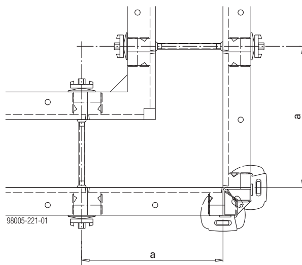
Vázlat: Framax Xlife sarokkialakítás
