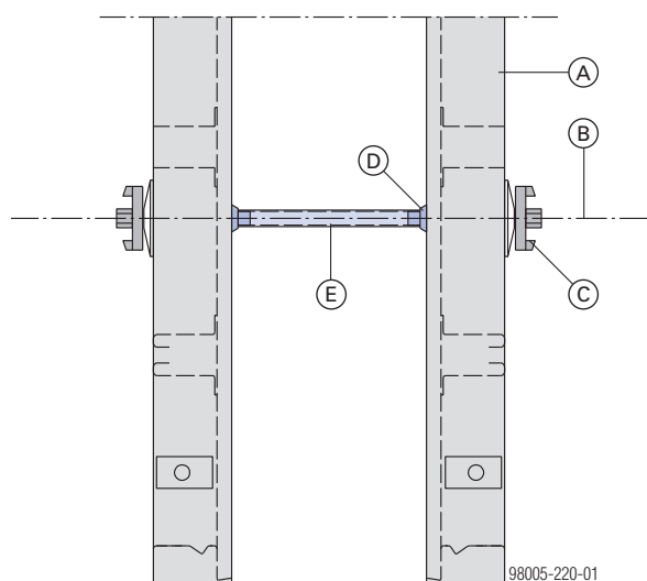
Ankerátkötés vázlata:
