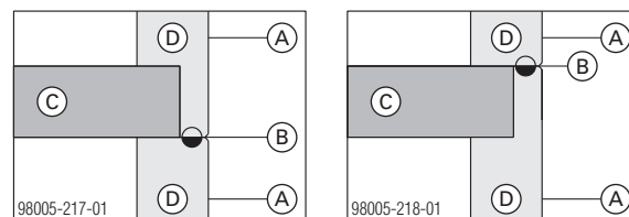
Bal oldali ábra: Födém alsó él munkahézag
