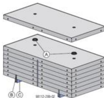
A Framax Xlife plus dubbelkonus resp. Framax Xlife plus dubbelkonus I
