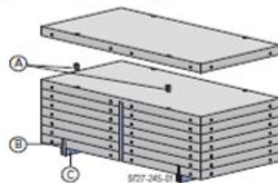
A Framax dubbelkonus
