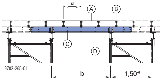
Kuva: Tukitorni Aluxo ja yläraakenne
