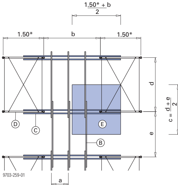
Pohjapiirros Tukitorni Aluxo ja yläraakenne
