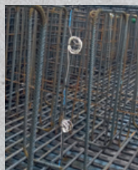
De kabelsensor is uitgerust met drie meetpunten en wordt, voordat het beton wordt gestort, aan de wapening bevestigd.
