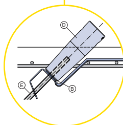
Spännstagshållare med ingjutningsgods Sida 7
