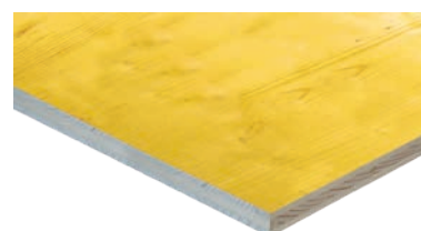
Doka 3-skiktsskiva 3S basic 21mm
