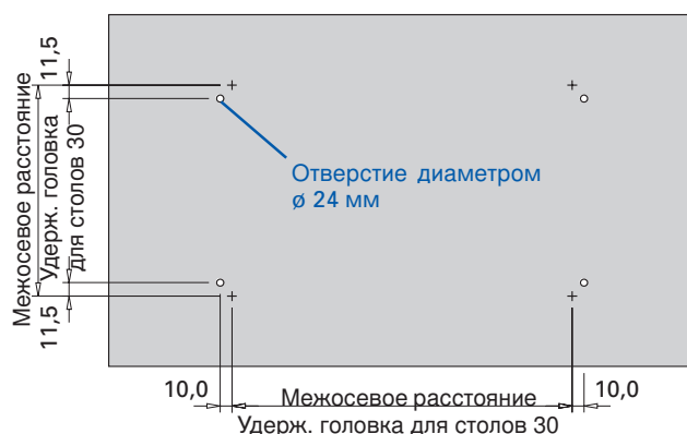
Схема сверлений (стол Dokaflex сверху)
