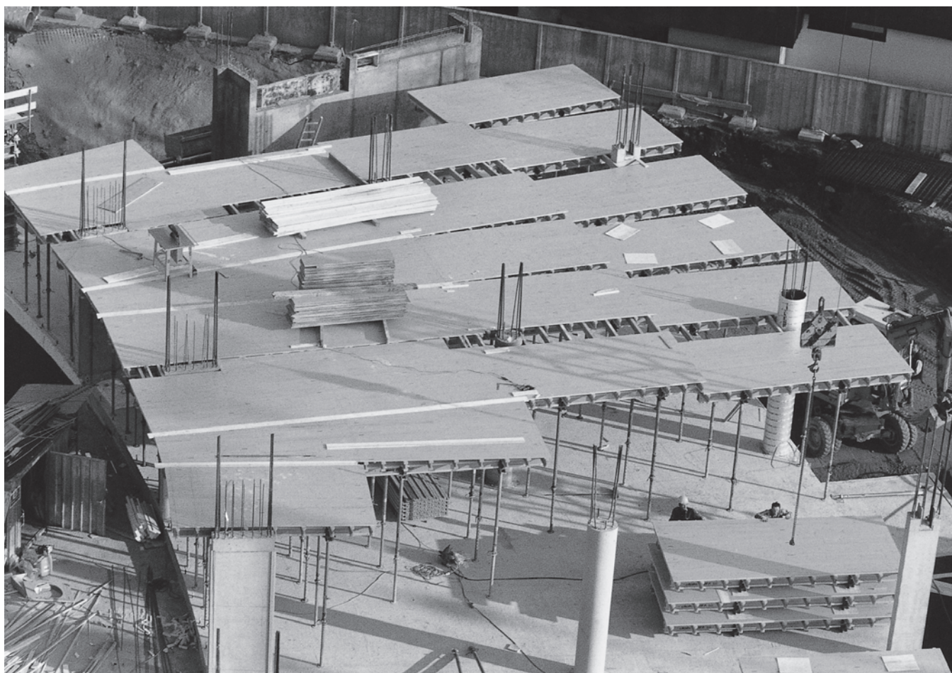
Строительная площадка: Chirurgie West, г. Зальцбург
