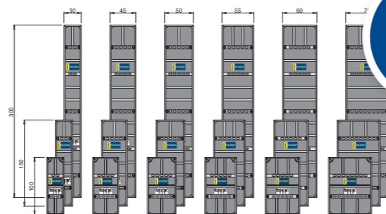
Semplice adeguamento alla costruzione grazie al logico sistema modulare a passi di 15 cm
