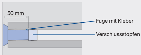
Sichbetonstopfen eingeklebt
