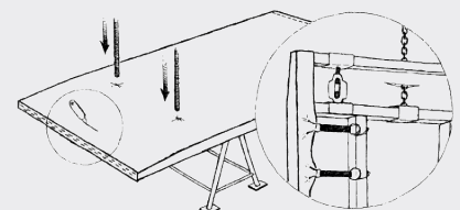
Festspannen über die Schalung mit Spannhaken.
